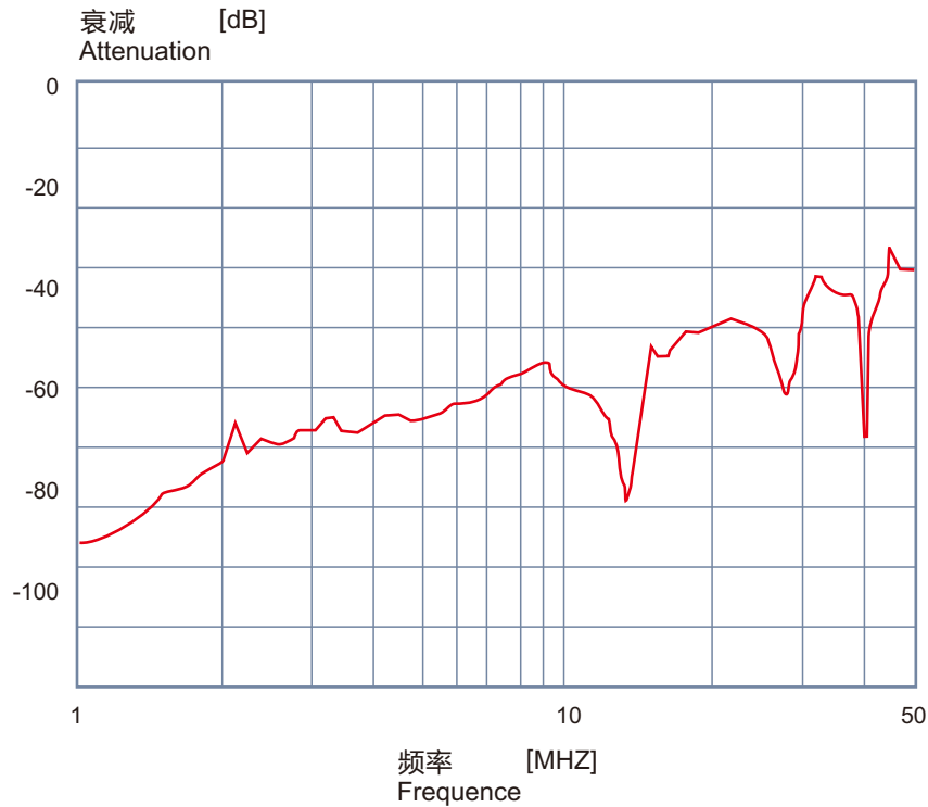
符合DIN 47250-6标准的衰减曲线 适用于电缆连接器
